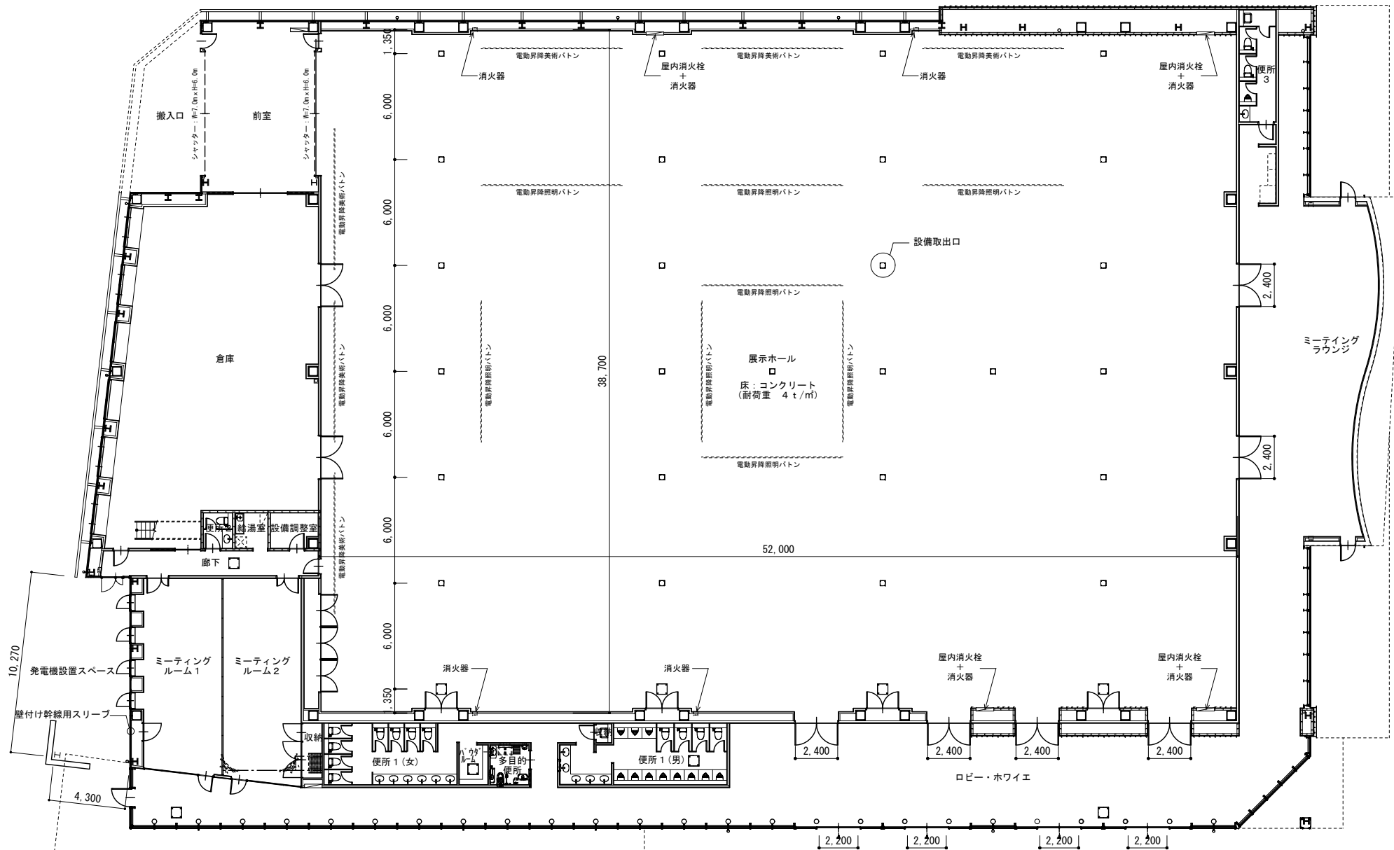
※本図面は現時点での図面であり、変更の可能性があります。 展示会館平面図 S=1:300 (A4版)
